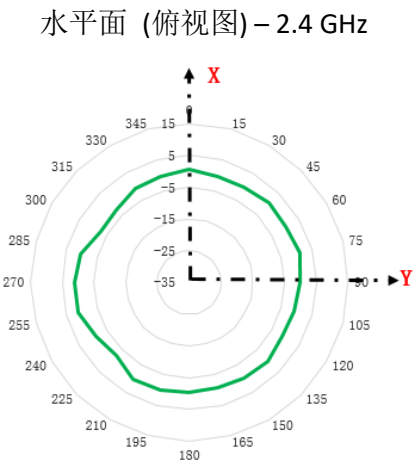
图 1. AP361-L 天线向量图
